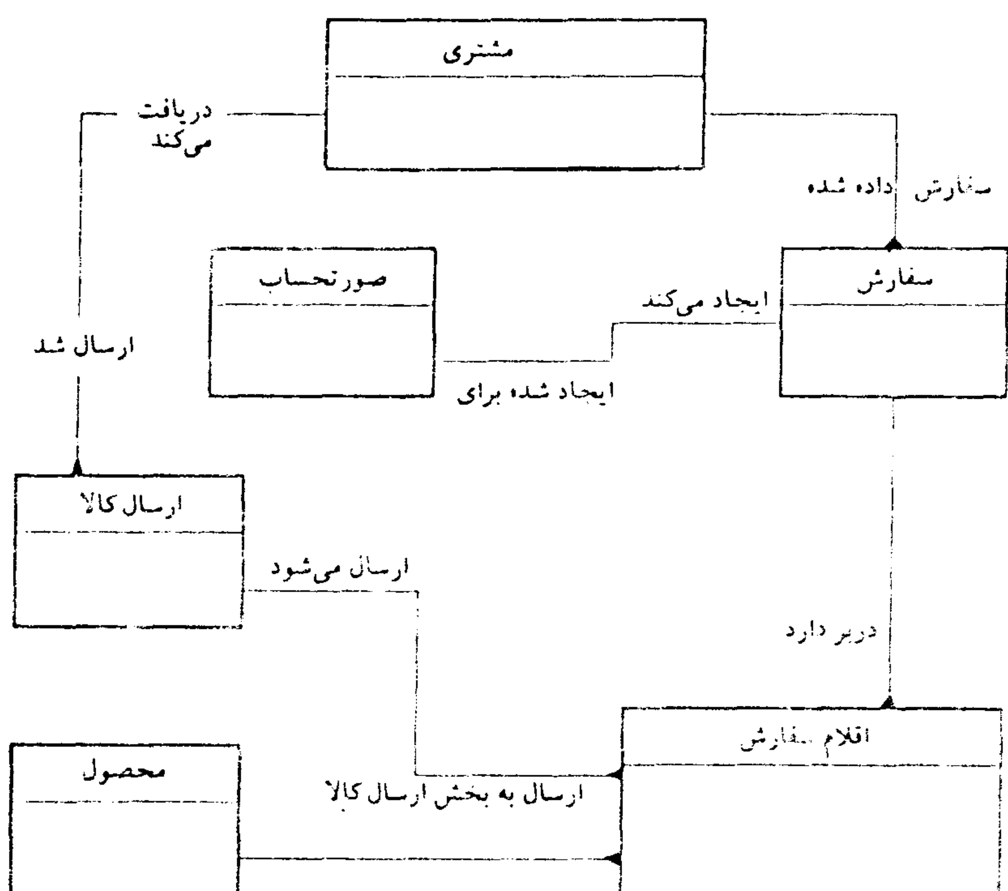
شکل شماره ۲ - مدل مفهومی اطلاعات شرکت پخش عدالت گستر
